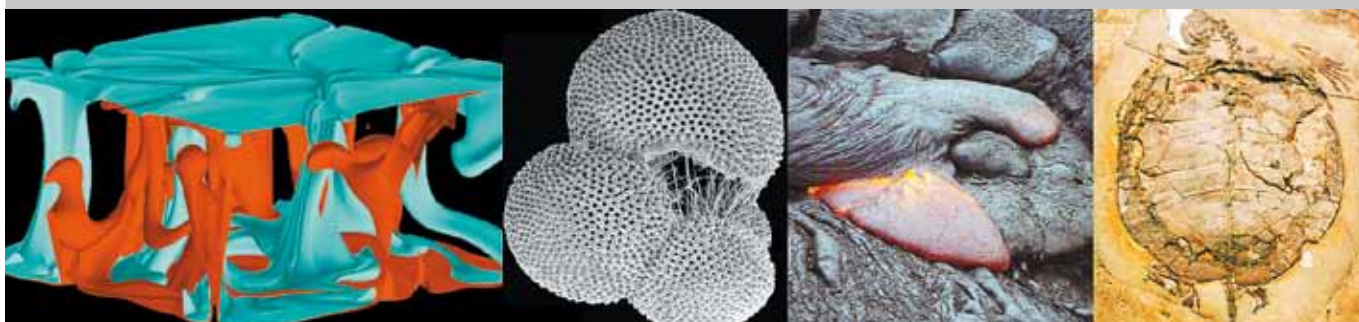
Convection dans le manteau
